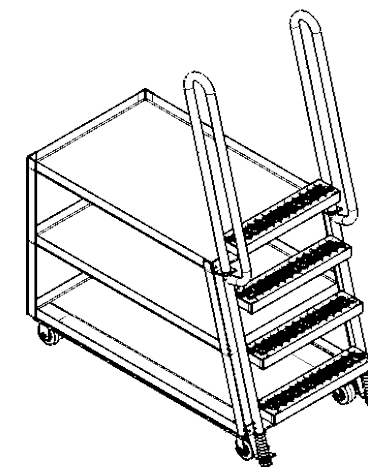
ISOMETRIC VIEW SCALE: 1:32
