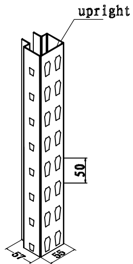
Upright
